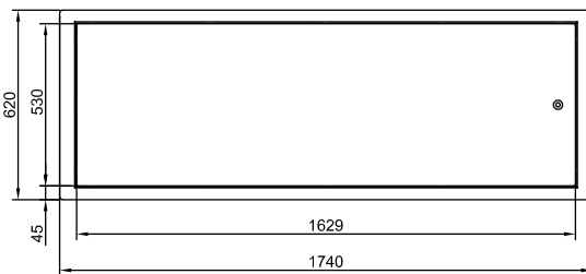
Boven aanzicht
